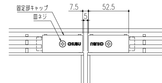
平面詳細図（ボルト固定部） S=1/2
